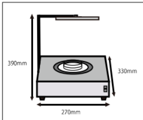
寸法
