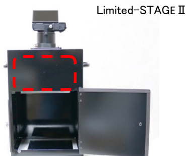
落射撮影 (キャビネット内 上部前後より照射)
